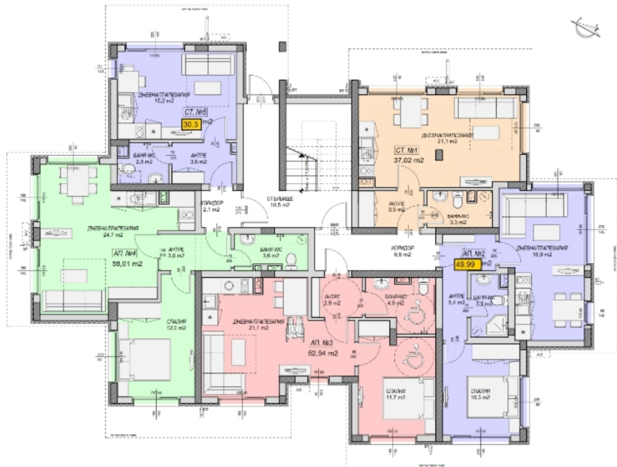
РАЗПРЕДЕЛЕНИЕ ПАРТЕР НА КОТА ±0,00
