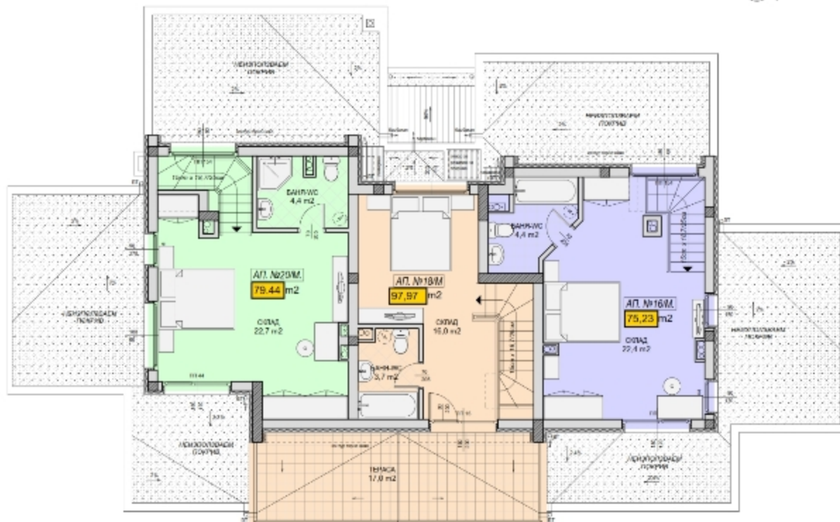
РАЗПРЕДЕЛЕНИЕ ТЕРАСОВИДЕН ЭТАЖ НА КОТА +11,20
